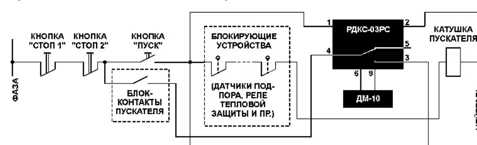
Рис. 5. Пример включения РДКС-03 в схему блокировки автономного конвейера.
