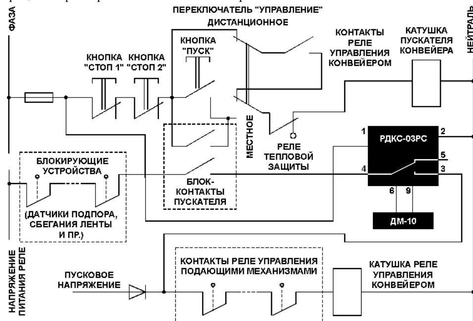
Рис. 6. Пример включения РДКС-03 в схему группового запуска линии.
